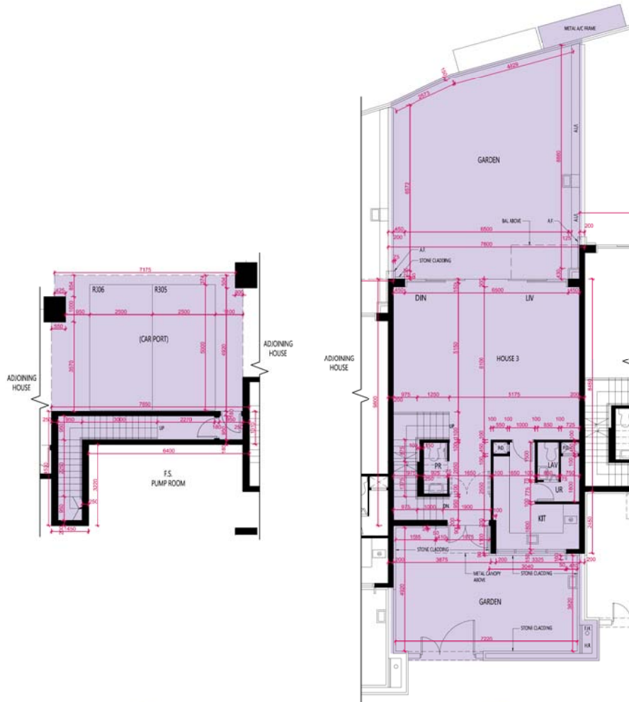
B/F 地庫
