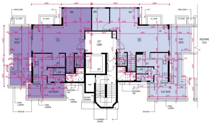
5/F 5樓
