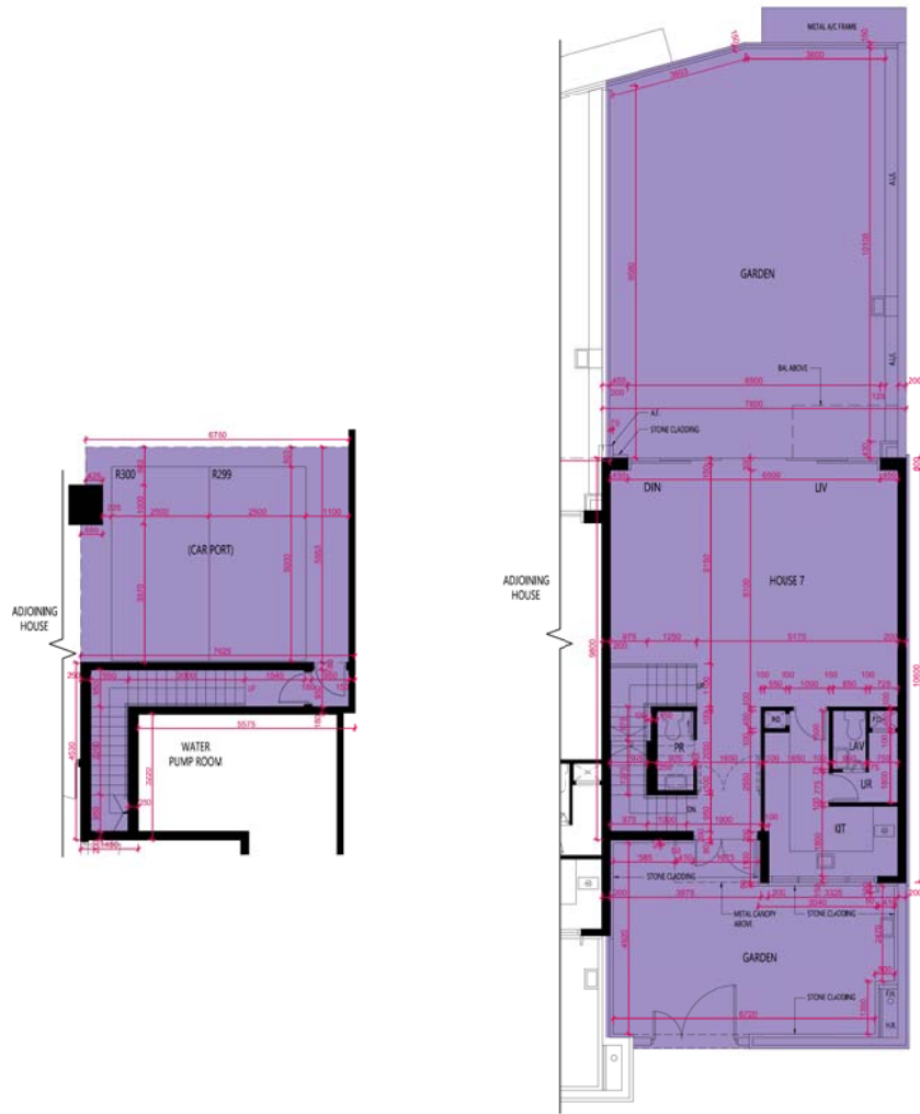
B/F 地庫
