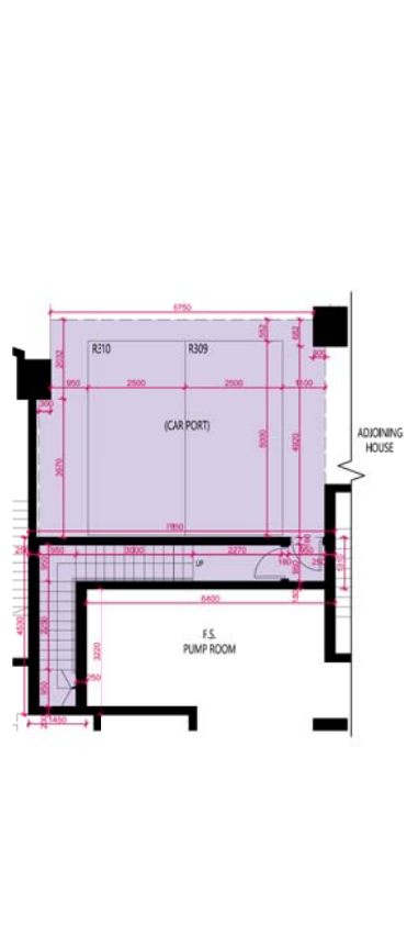
B/F 地庫
