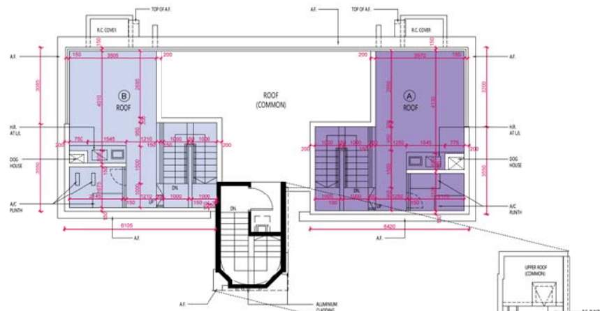
ROOF 天台
