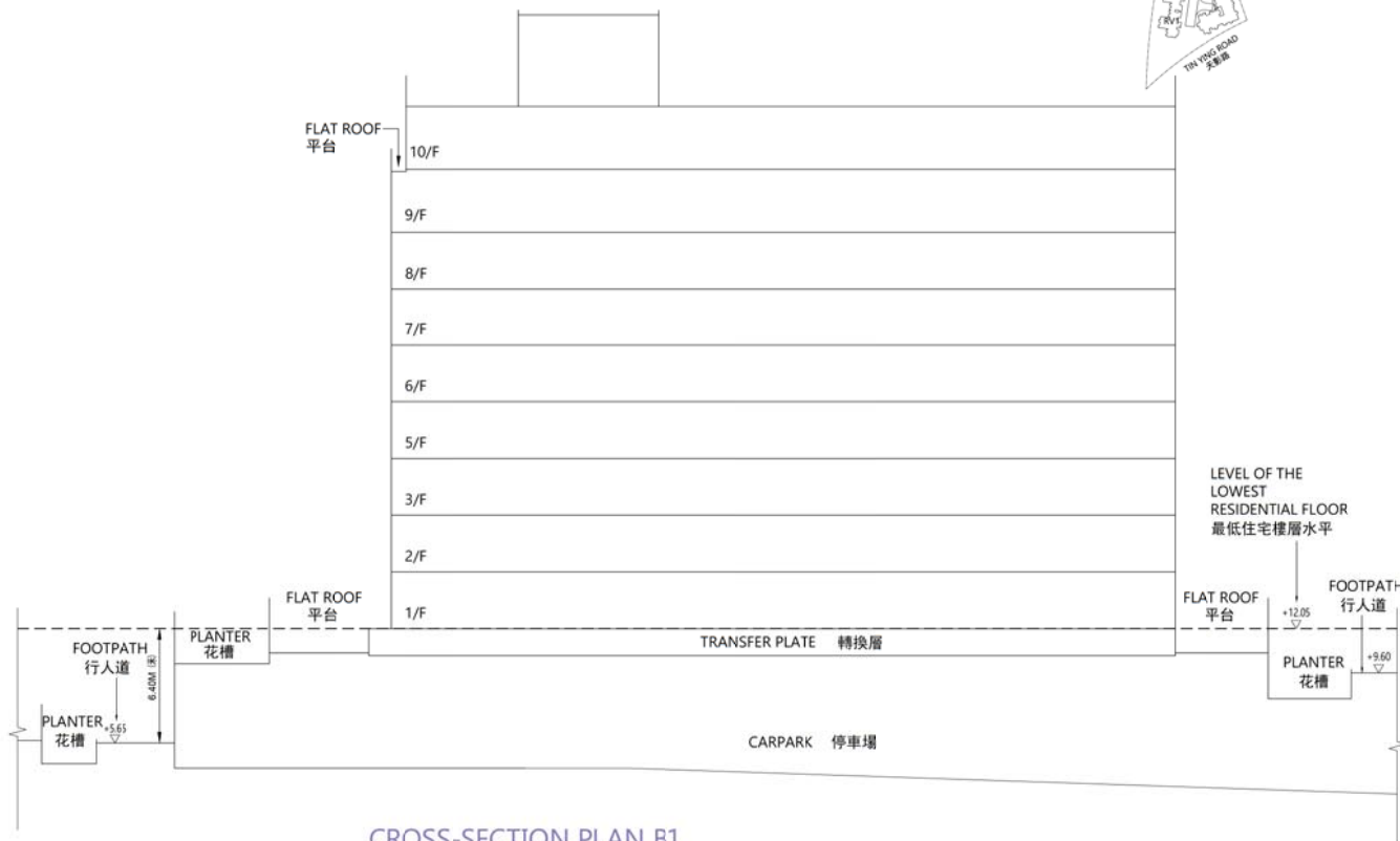
CROSS-SECTION PLAN B1 橫截面圖 B1
