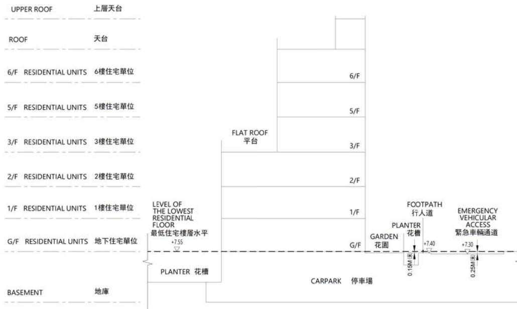
CROSS-SECTION PLAN C1 橫截面圖 C1
