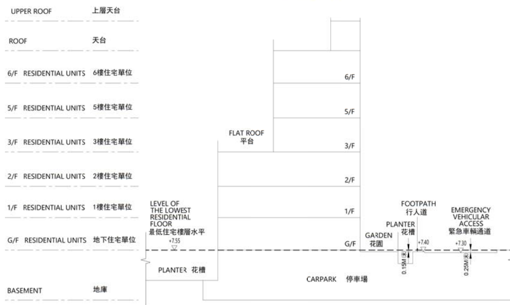
CROSS-SECTION PLAN D1 橫截面圖 D1
