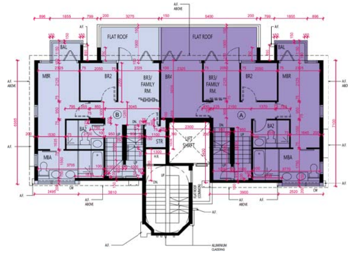
6/F 6樓
