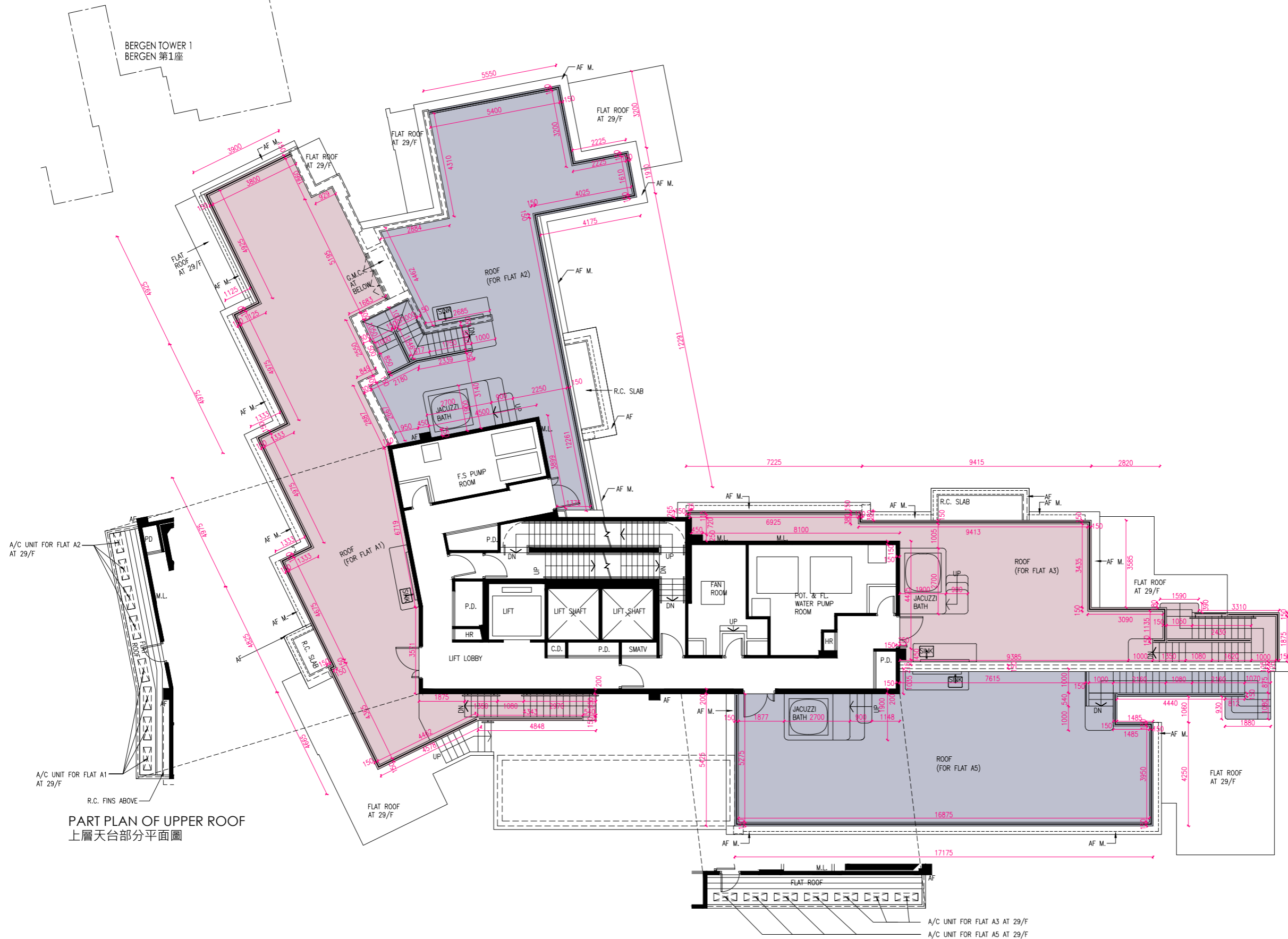
PART PLAN OF UPPER ROOF 上層天台部分平面圖
