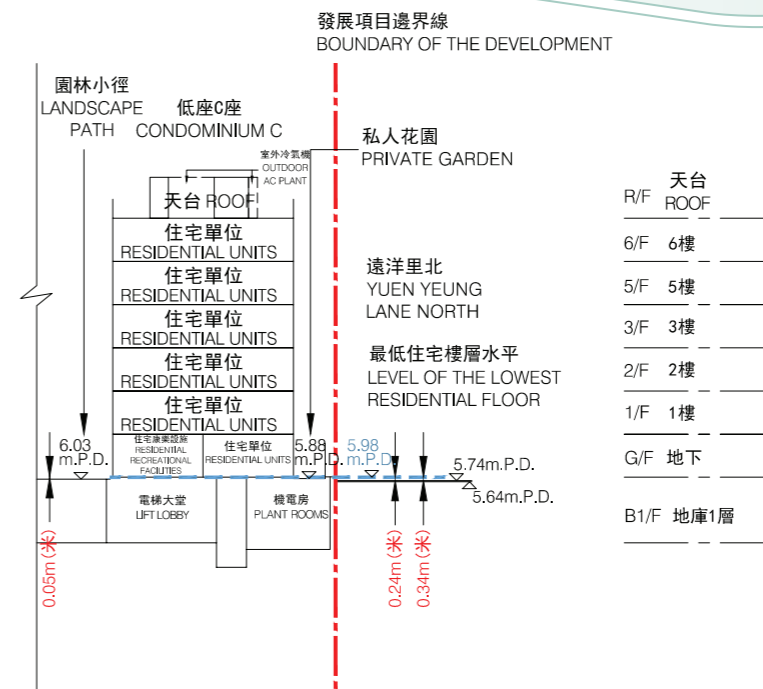
橫截面圖 F-F' Section F-F'
