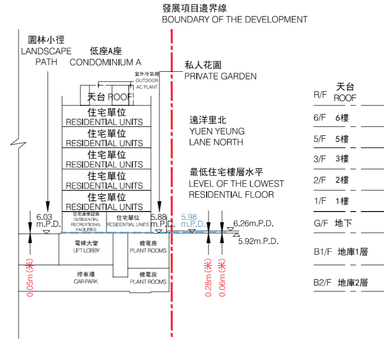
橫截面圖 D-D' Section D-D'
