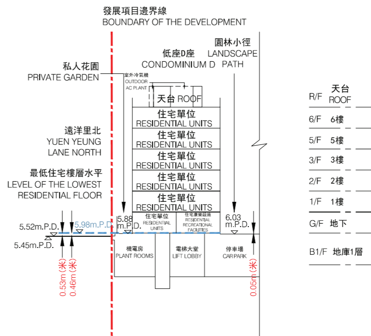
橫截面圖 G-G' Section G-G'
