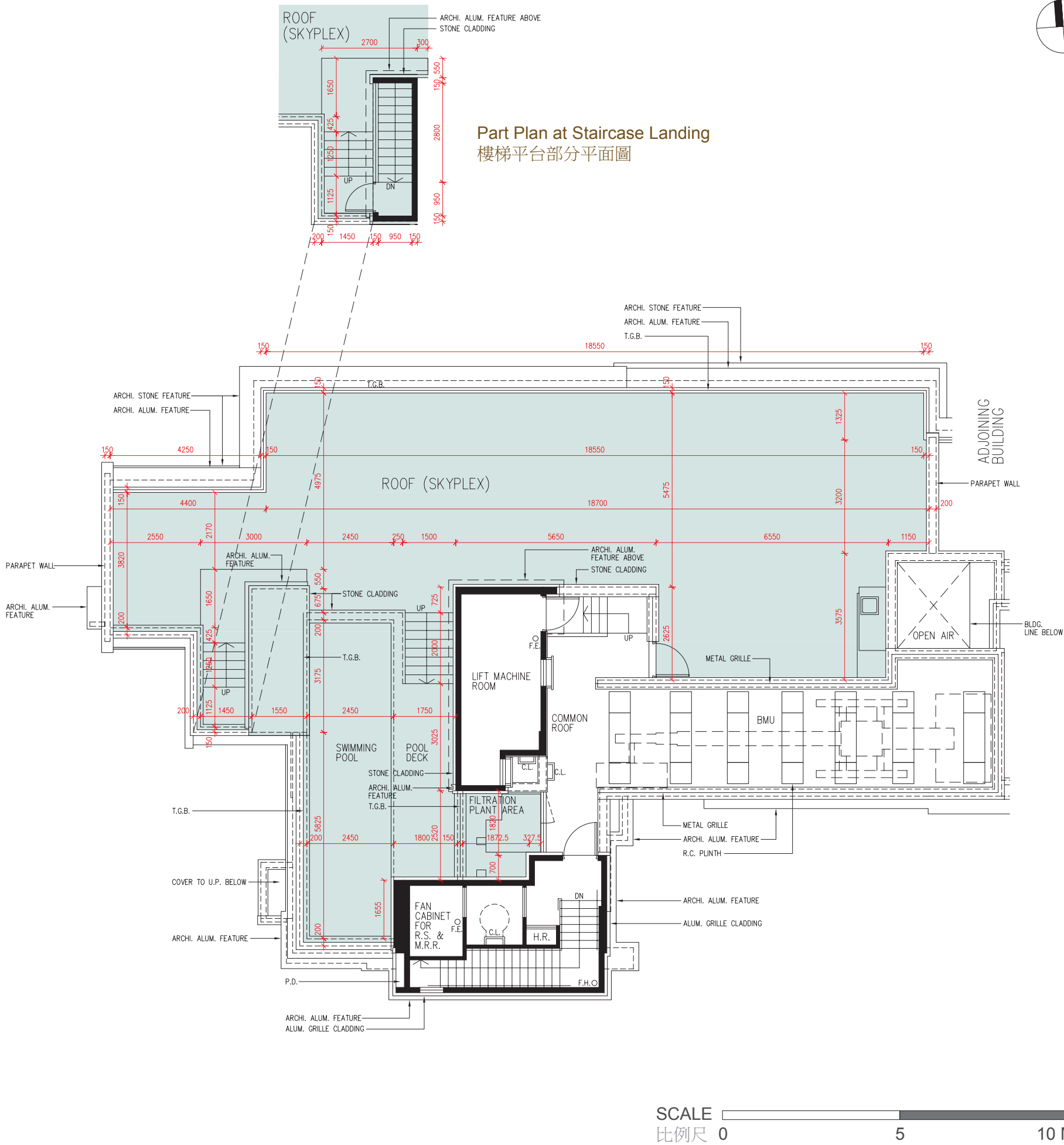
Alpex III Roof Plan 天台平面圖
